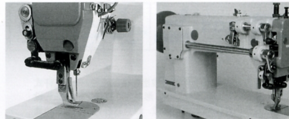
GC0318-1A 上下复合送料厚料平缝机
