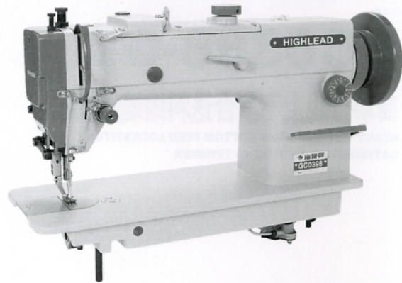
GC0398-1 上下复合送料厚料平缝机
