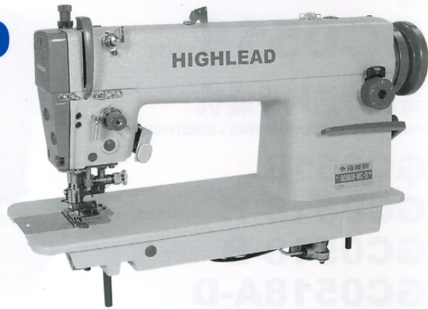
GC0518-MC 高速针送料侧切刀平缝机
