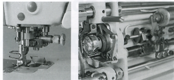
GC0518-MC 高速针送料侧切刀平缝机
