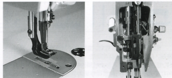
GC0618-1 综合送料厚料平缝机
