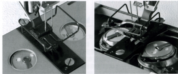
GC20568-MDZ 直驱式微油自动剪线高速双针平缝机
