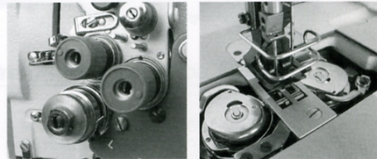
GC20638-D 自动剪线综合送料针杆离合双针平缝机
