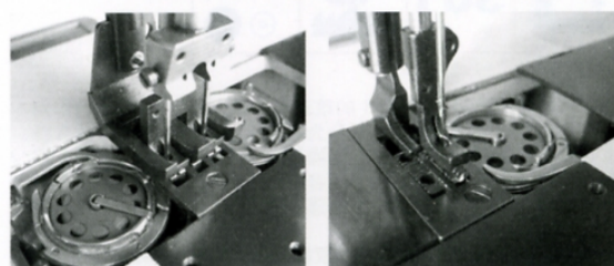
GC20698-6 综合送料双针厚料平缝机
