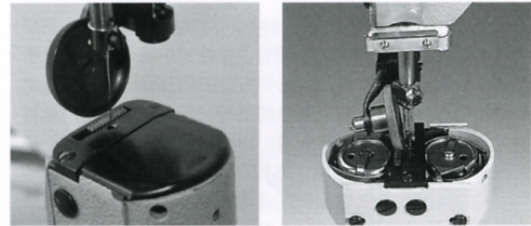
GC24018-1 立柱式双针平缝机
