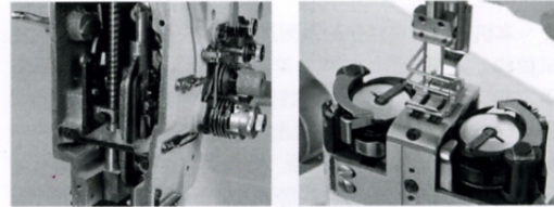
GC24518-2 立柱式针送料双针平缝机
