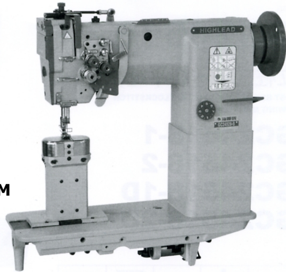
GC24528-B 立柱式针杆离合双针平缝机
