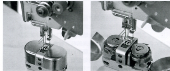
GC24528-B 立柱式针杆离合双针平缝机
