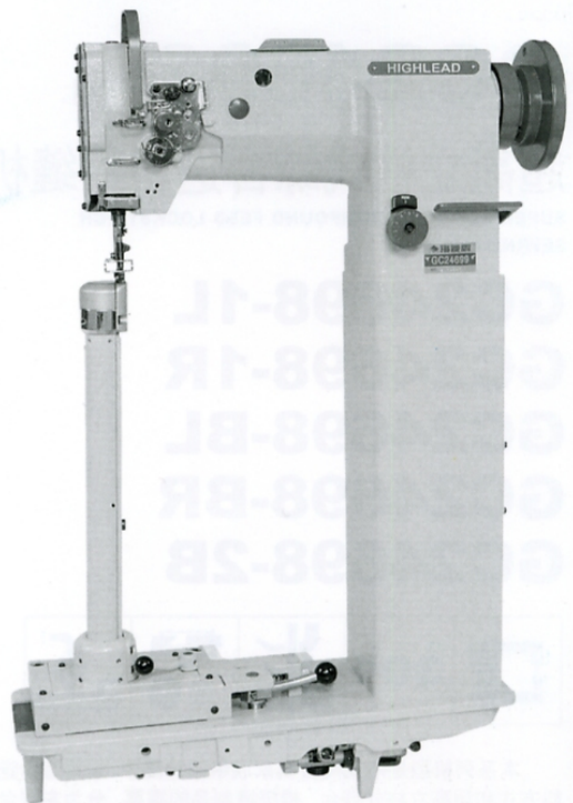
GC24699 可倾式超高立柱综合送料平缝机
