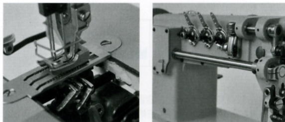
GK0318-2 上下复合送料链式平缝机
