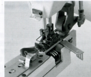
GK3088-3T 筒式卷接缝纫机
