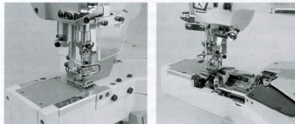
GK600-4 高速三针小方筒式绷缝机
